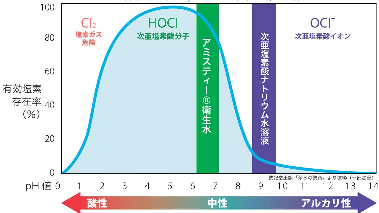
遊離有効塩素の pH による存在比率の変化
