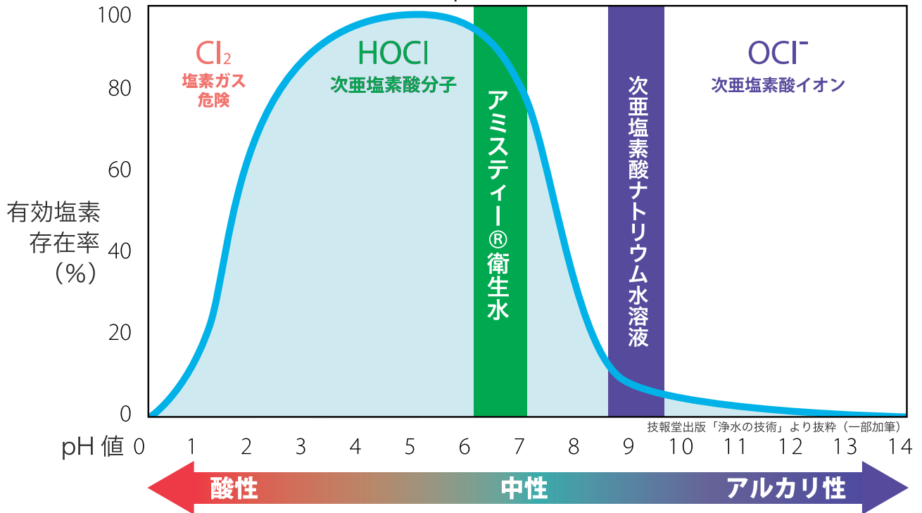
遊離有効塩素の pH による存在比率の変化
